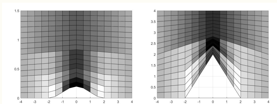
Рис. 11.1: Разностная сетка и распределение показателя преломления в анизотропном материале (а) произвольное искажение границы, (б) линейное искажение границы.
